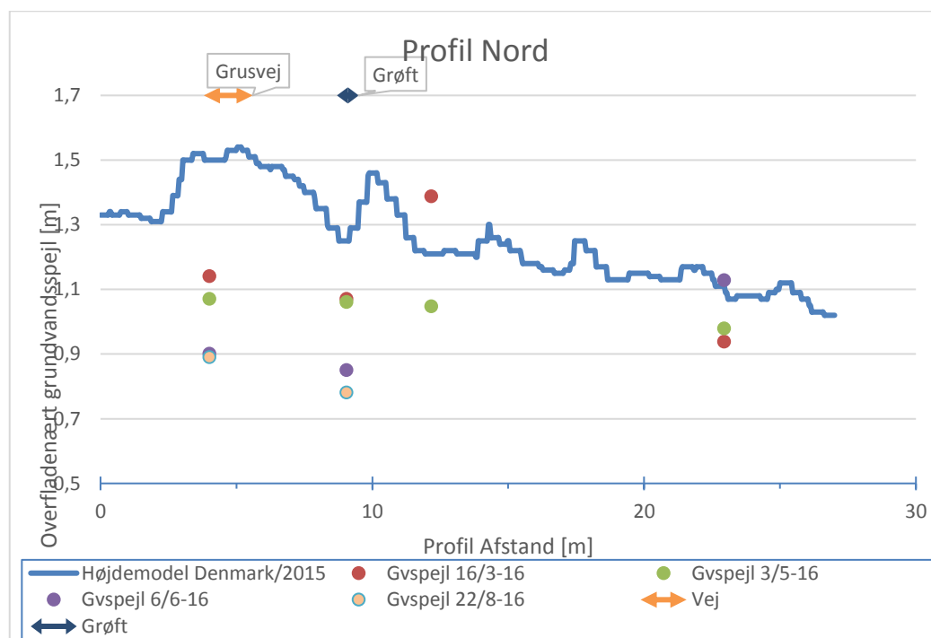
Figur 5-10. Terrænprofil og observerede vandspejl i etablerede boringer på profil Nord.
